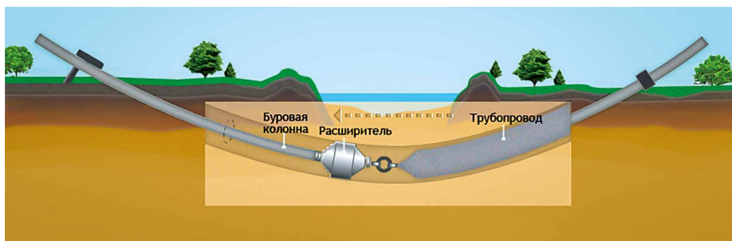
Схема работ методом наклонно-направленного бурения
