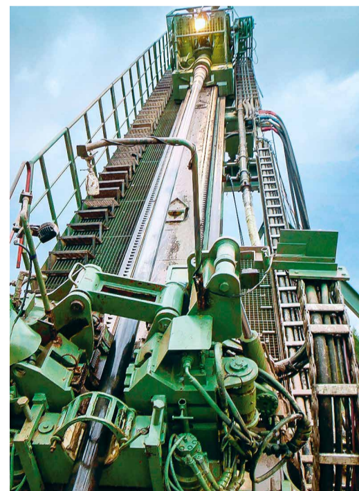
Установка для наклонно-направленного бурения
