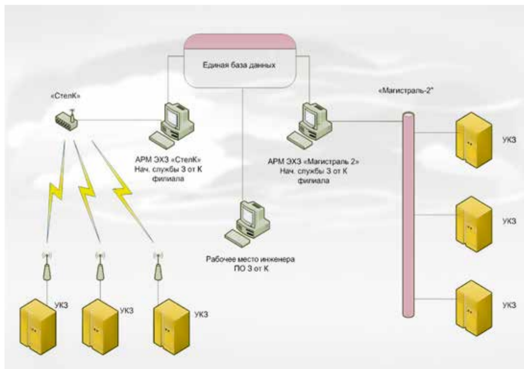
Предлагаемая схема организации системы телемеханики средств ЭХЗ Общества
