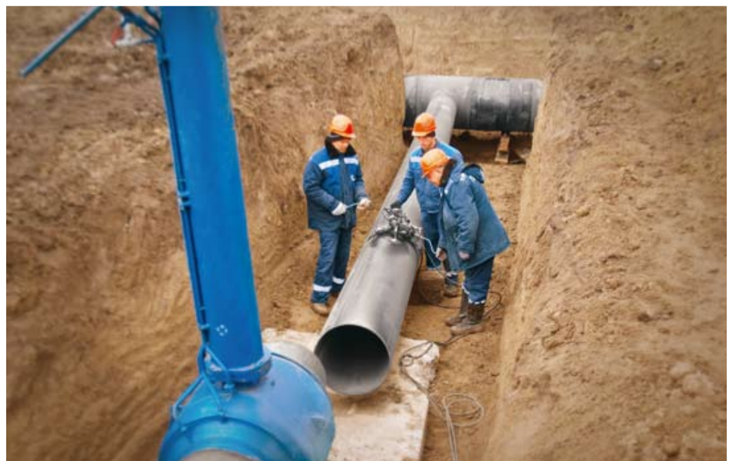
Врезка крана
